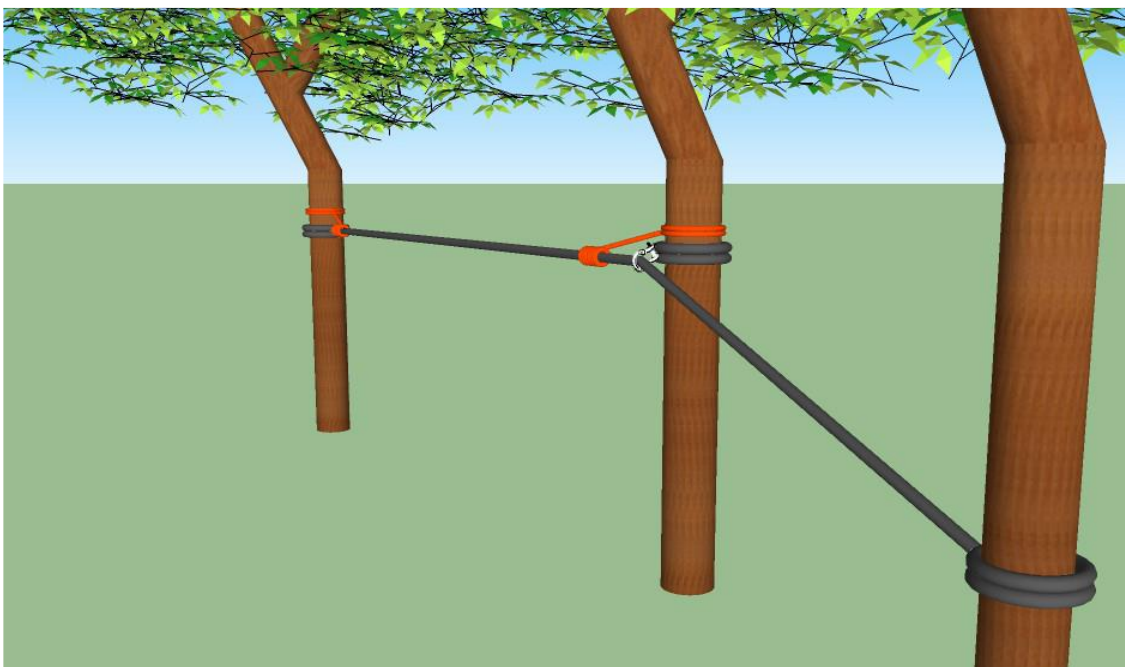
Hoofdlijn met kritisch omliep punt, hier is het veiligheidstouw aangebracht
